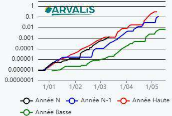
Rouille Jaune - Parcelle : Cas type BSV 2 NIORT, Station NIORT SOUCHE - Date de semis 25/11, Année Haute 2014 - Année Basse 2006
